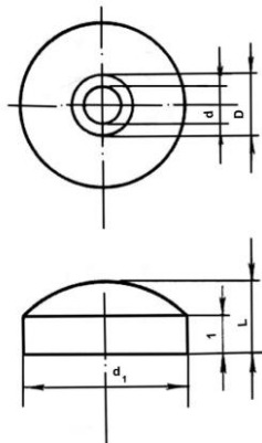
Рис. 1. Шаблон для определения достоинства пробоин
